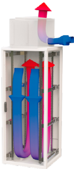
PRŮTOK VZDUCHU ROZVADĚČEM – COOLSPOT DX TM VERZE
