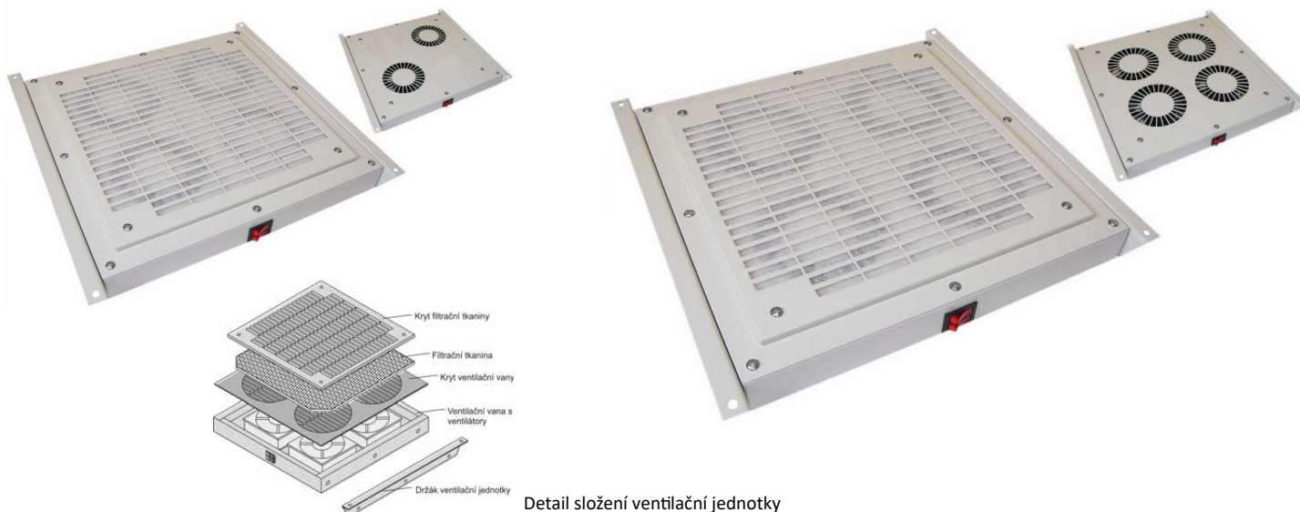
Detail složení ventilační jednotky
