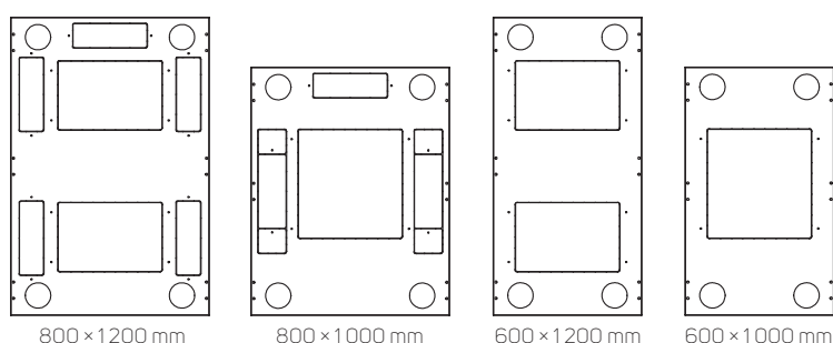
HORNÍ POHLED
