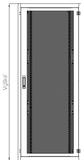
ZADNÍ POHLED
